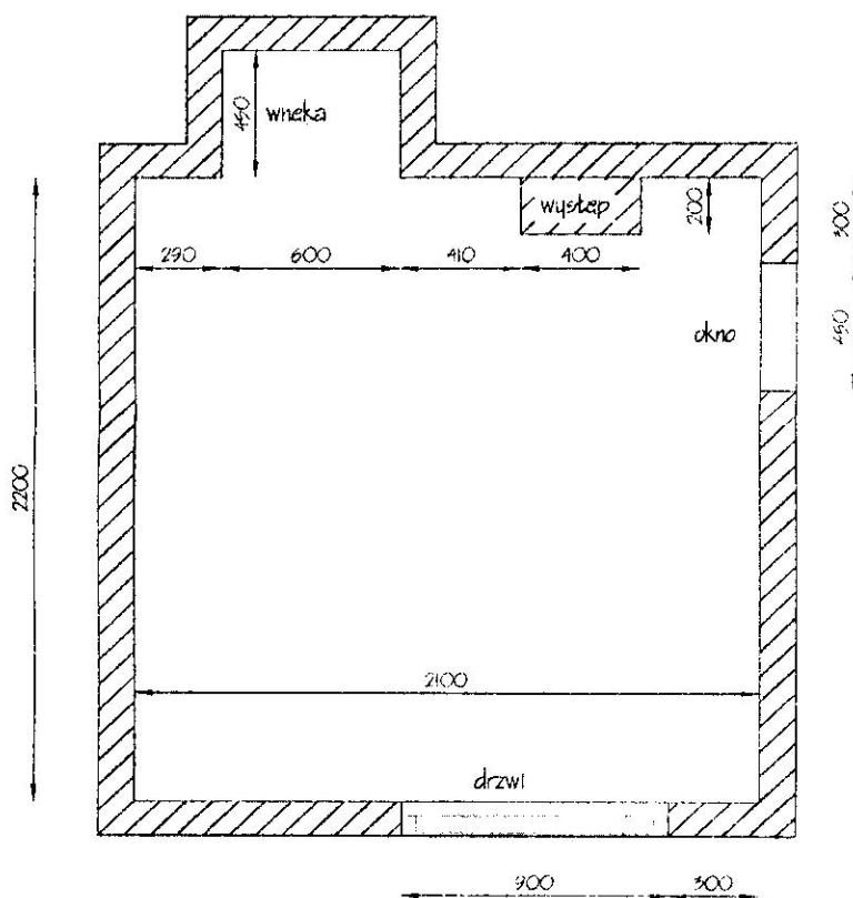
przykład prawidłowo wymiarowanego pomieszczenia [ mm ]
